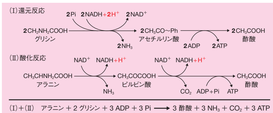
p48 図 5.3 スティックランド反応によるアミノ酸を基質とする発酵
