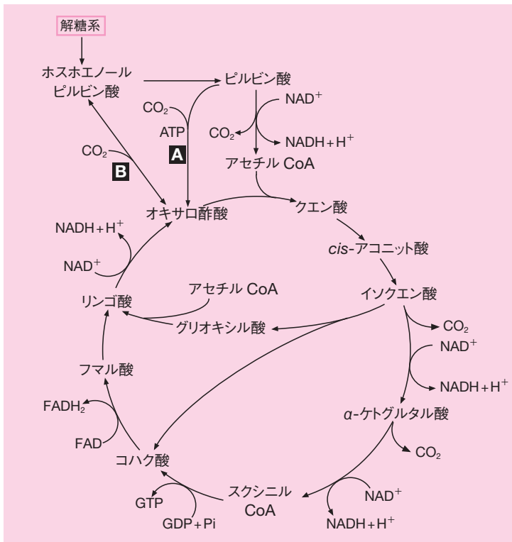
p49 図 5.5 クエン酸回路とそれに関連する補充反応とグリオキシル酸回路
